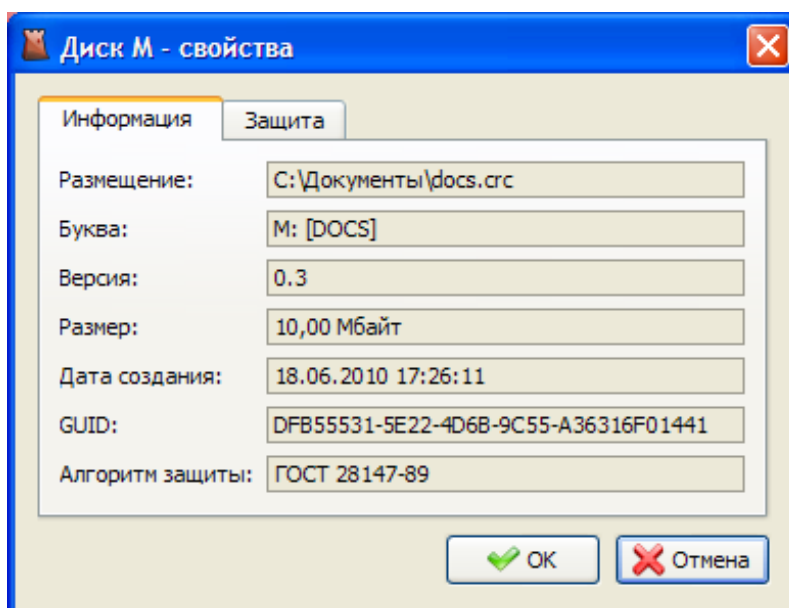
Рисунок 4.2. Диалог свойств криптообъекта - Информация
