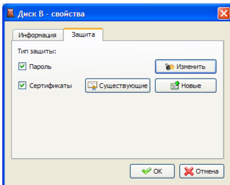
Рисунок 4.3. Диалог свойств криптообъекта - Защита
