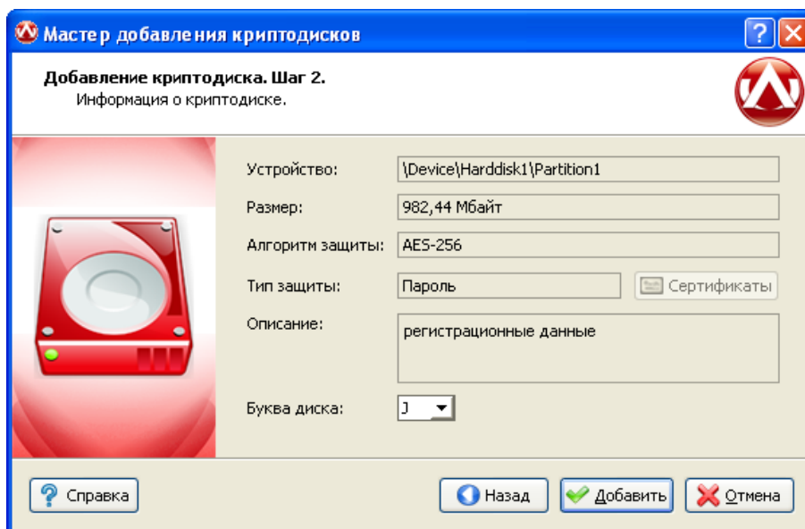
Рисунок 4.12. Мастер добавления криптокодисков. Сводная информация о криптодиске.
